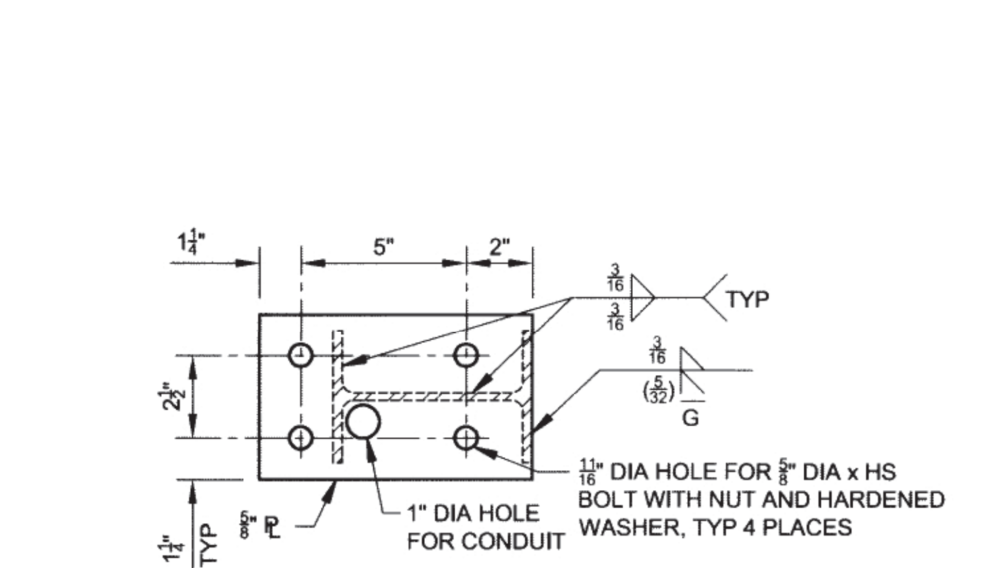
E1 SECTION A SCALE : 1 1/2" = 1'-0"
