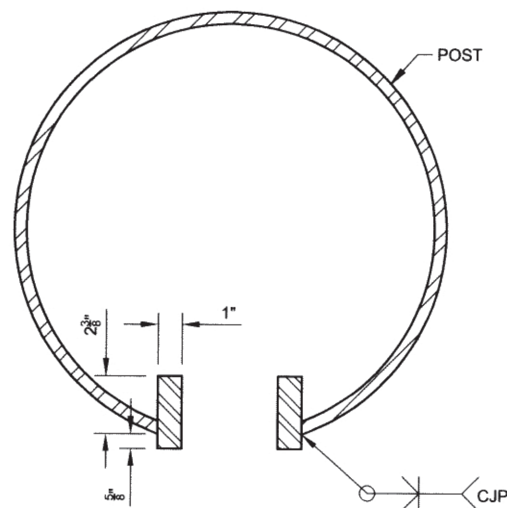
D1 SECTION A SCALE : 3" = 1'-0" S-4
