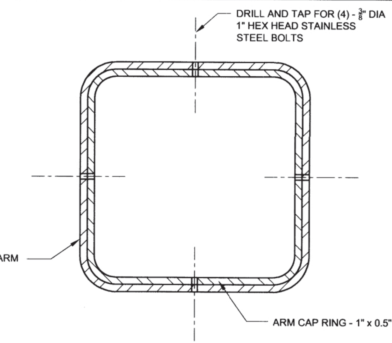
A6 SECTION D SCALE: 3" = 1'-0"
