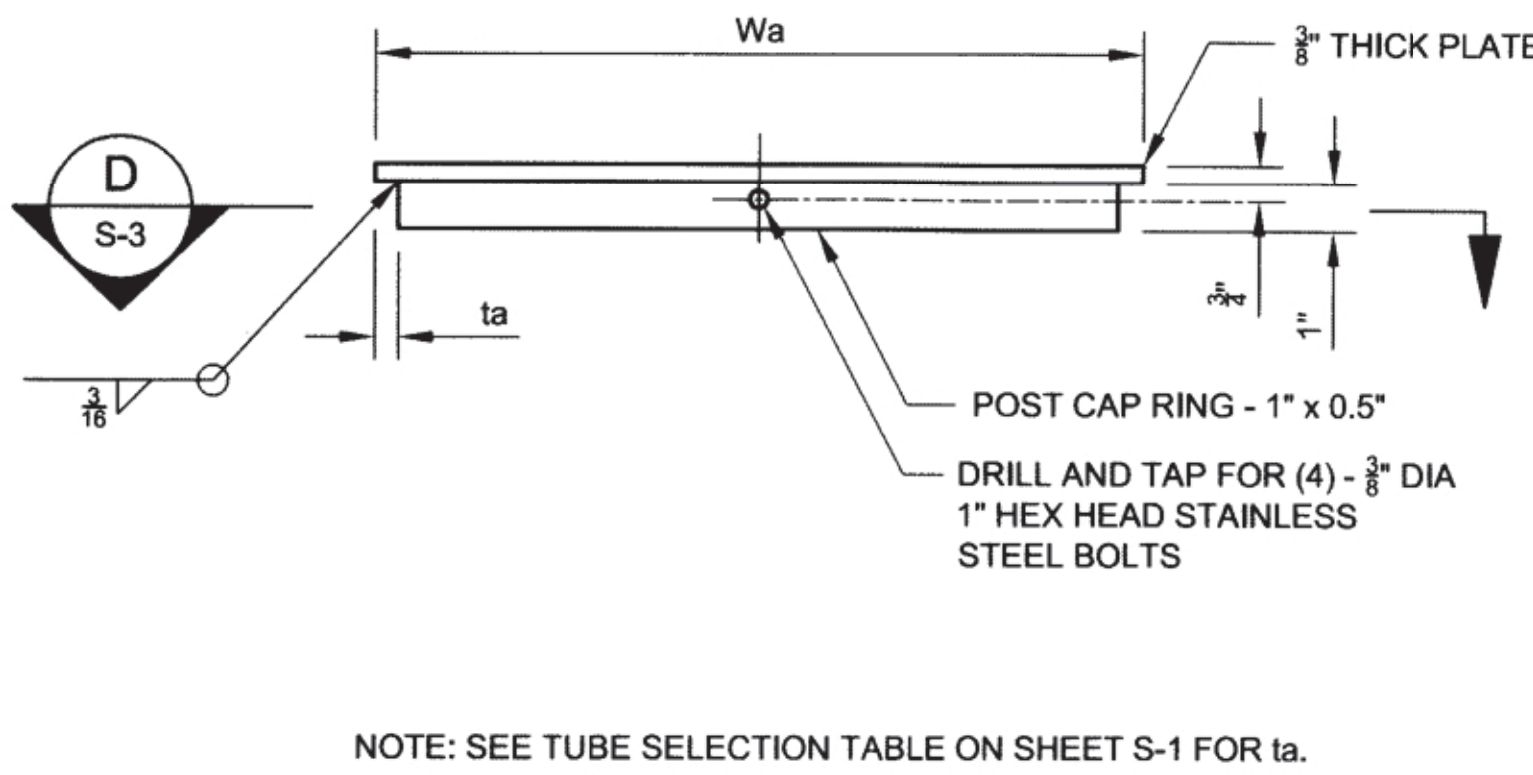
A1 ARM CAP DETAIL SCALE: 3" = 1'-0"
