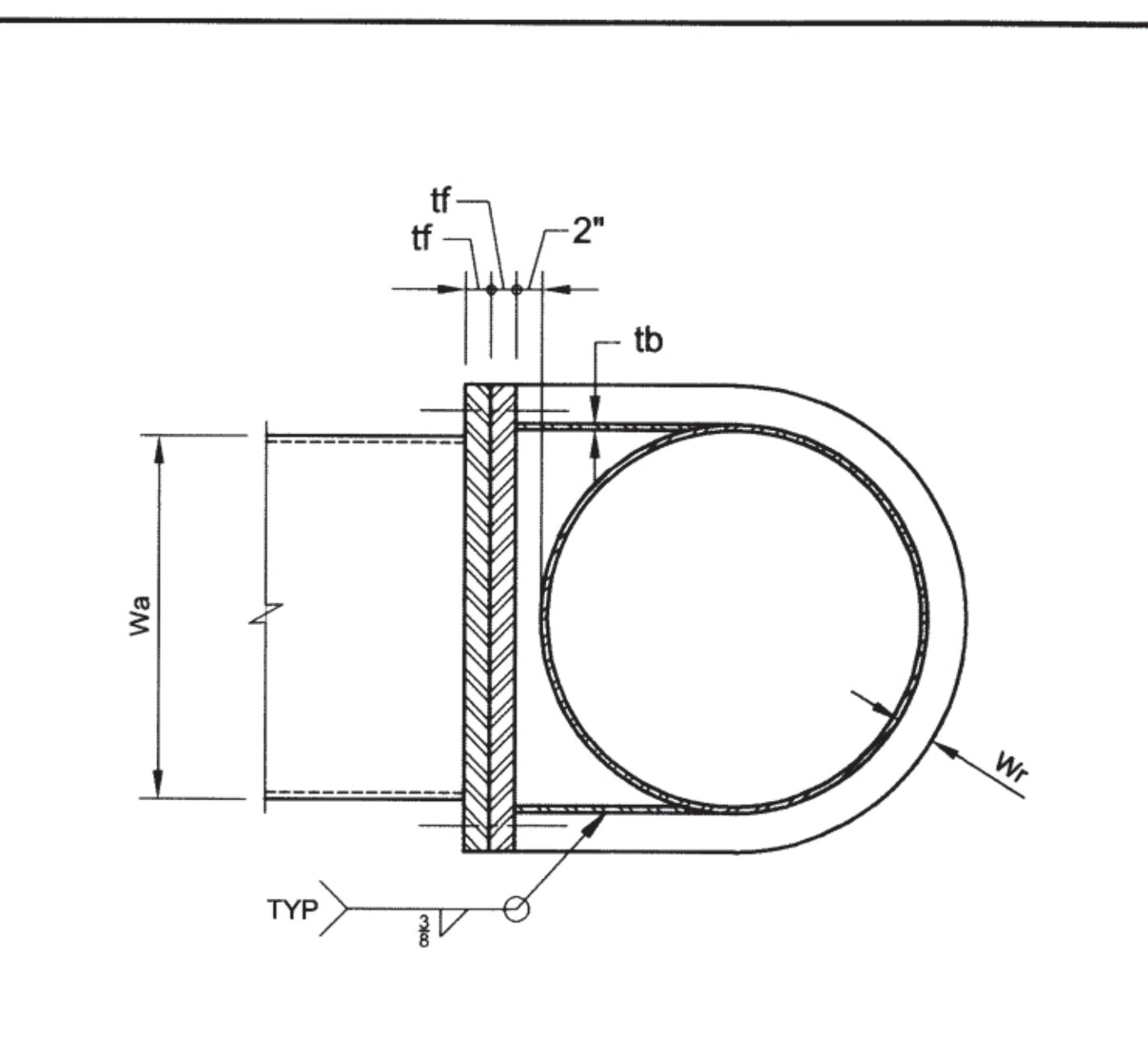
I13 SECTION B SCALE: 1" = 1'-0"
