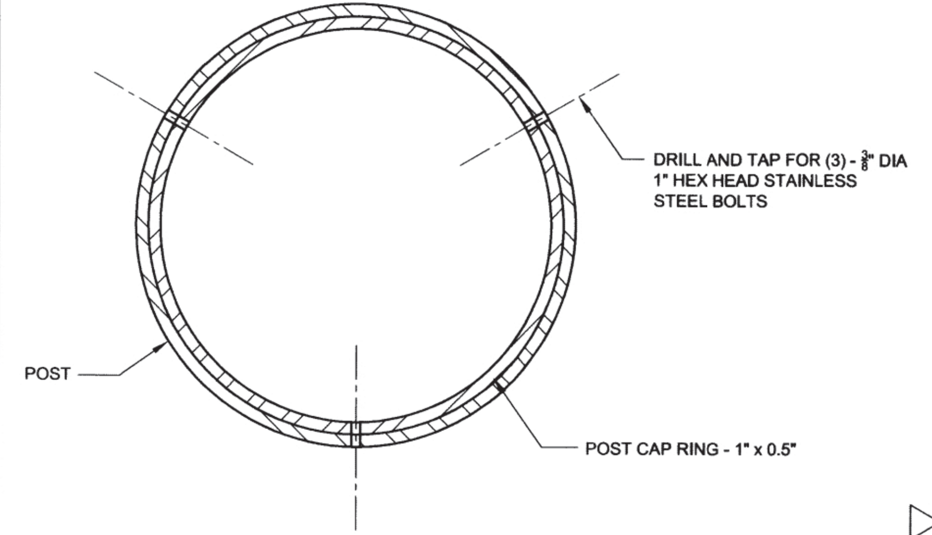
E12 SECTION C SCALE: 3" = 1'-0"
