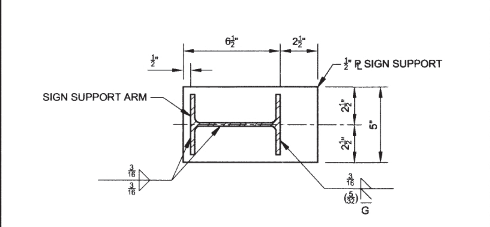
E13 SECTION C SCALE : 3" = 1'-0"
