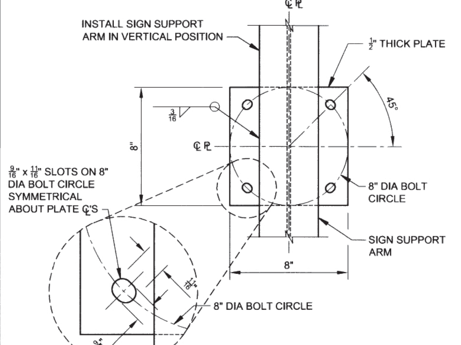
A5 SECTION E SCALE : 3" = 1'-0"
